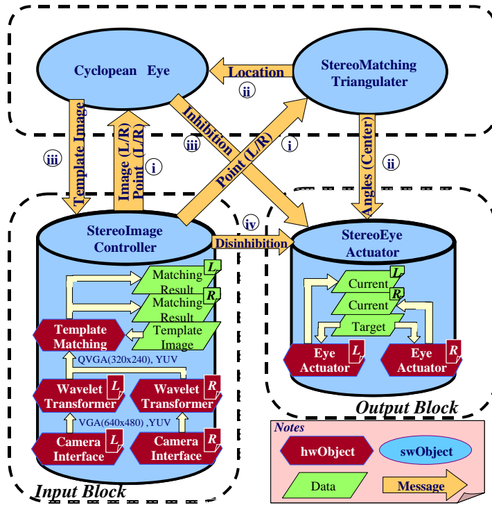
第2図 hwObject / swObjectによるアプリケーション構成
