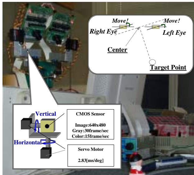
第3図 全体写真
